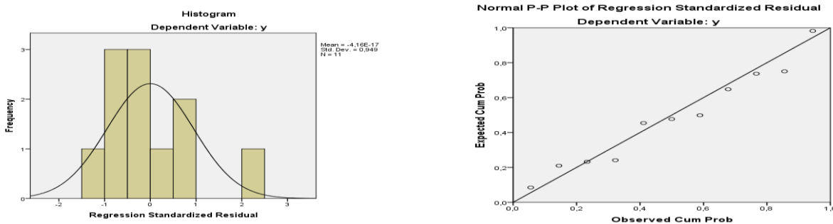
Gambar 4.2 gambar uji normalitas
