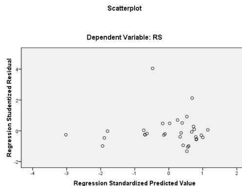
Gambar 2 Uji Heteroskedastisitas
