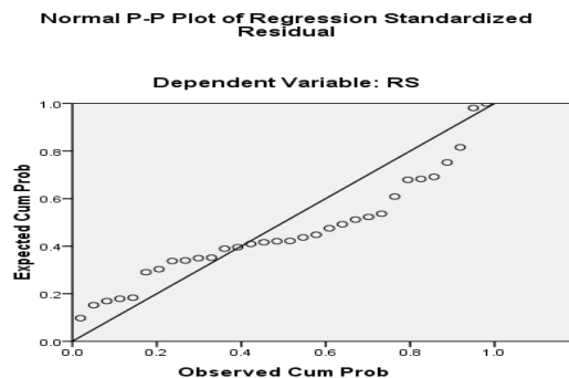
Gambar 1 Uji Normalitas
