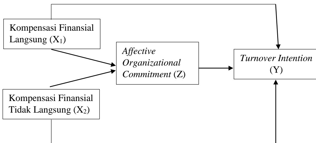
Gambar 3.1 Kerangka Konseptual
